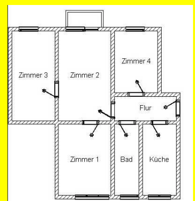
4 Raum Wohnung
